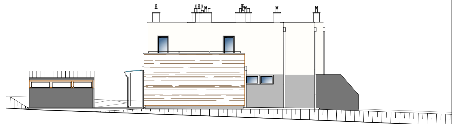
NORDWEST-ANSICHT REIHENHAUS 22-24
